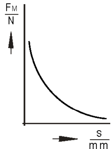
Bild 2: Magnetkraft-Hub-Kennlinie
