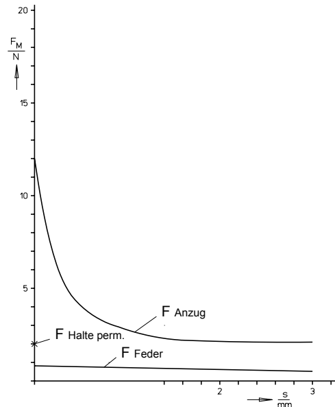
Bild 4: Magnetkraft-Hub-Kennlinie G BK P 017 K00 A02
