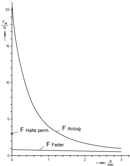
Bild 3: Magnetkraft-Hub-Kennlinie G BK P 017 K00 A01
