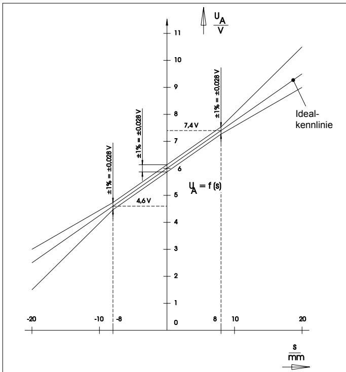
Bild 2: Kennlinie A WE X 020A01
