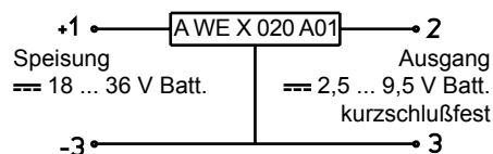
Bild 4: Blockschaltplan A WE X 020 A01
