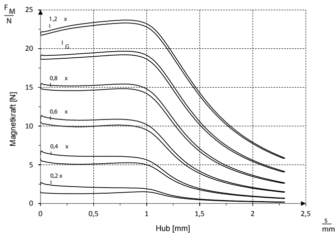
Bild 3: Magnetkraft-Hub-Kennlinie
