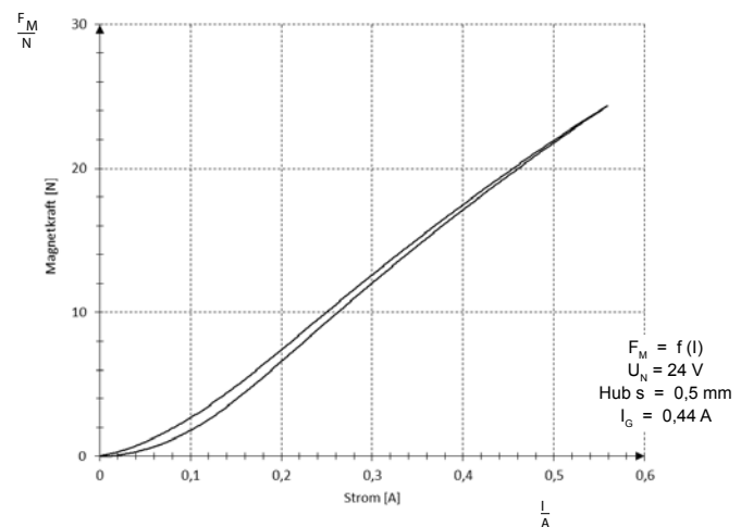
Bild 4: Magnetkraft-Strom-Kennlinie bei konstantem Hub
